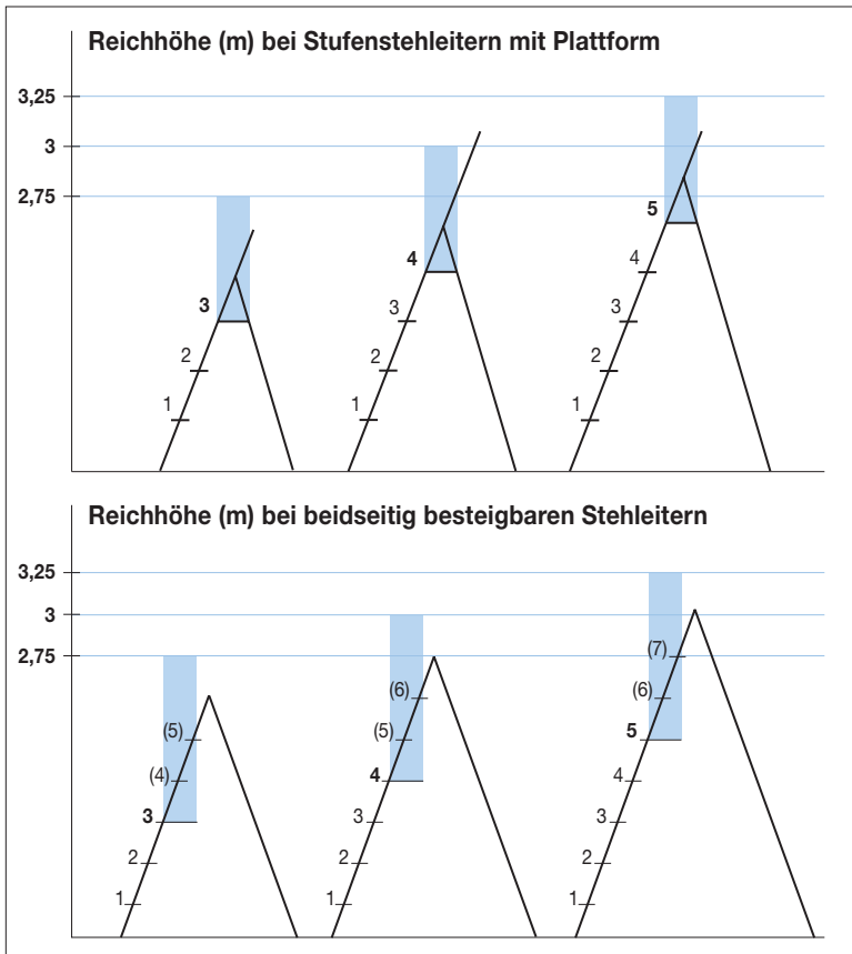
Bild 39: Reichhöhen
