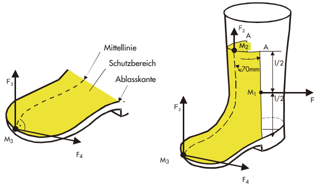
Bild 10 Gamasche mit Mindestschutzbereich
