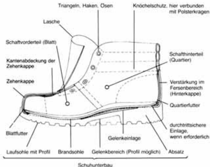
Bild 1: Beispiele für Bestandteile eines Schuhs
